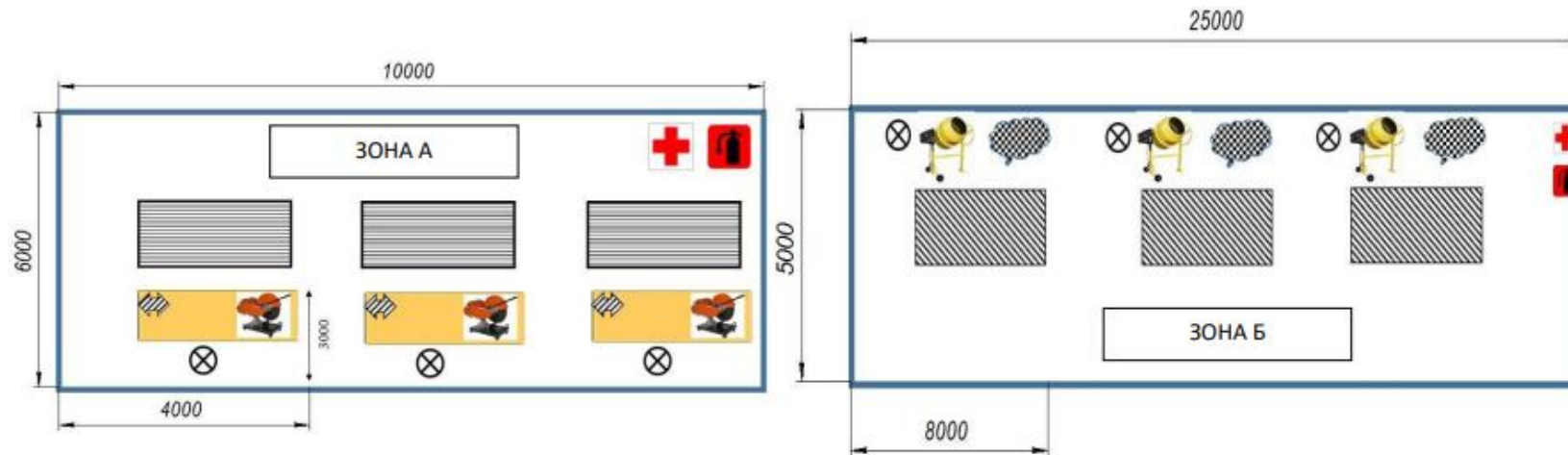
Примерный план застройки площадки ДЭ ПУ, проводимого в рамках ГИА
