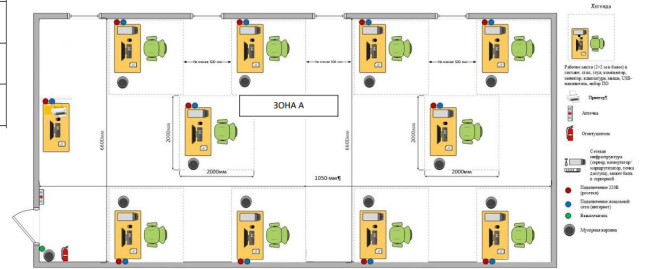
Примерный план застройки площадки ДЭ, проводимого в рамках ПА
